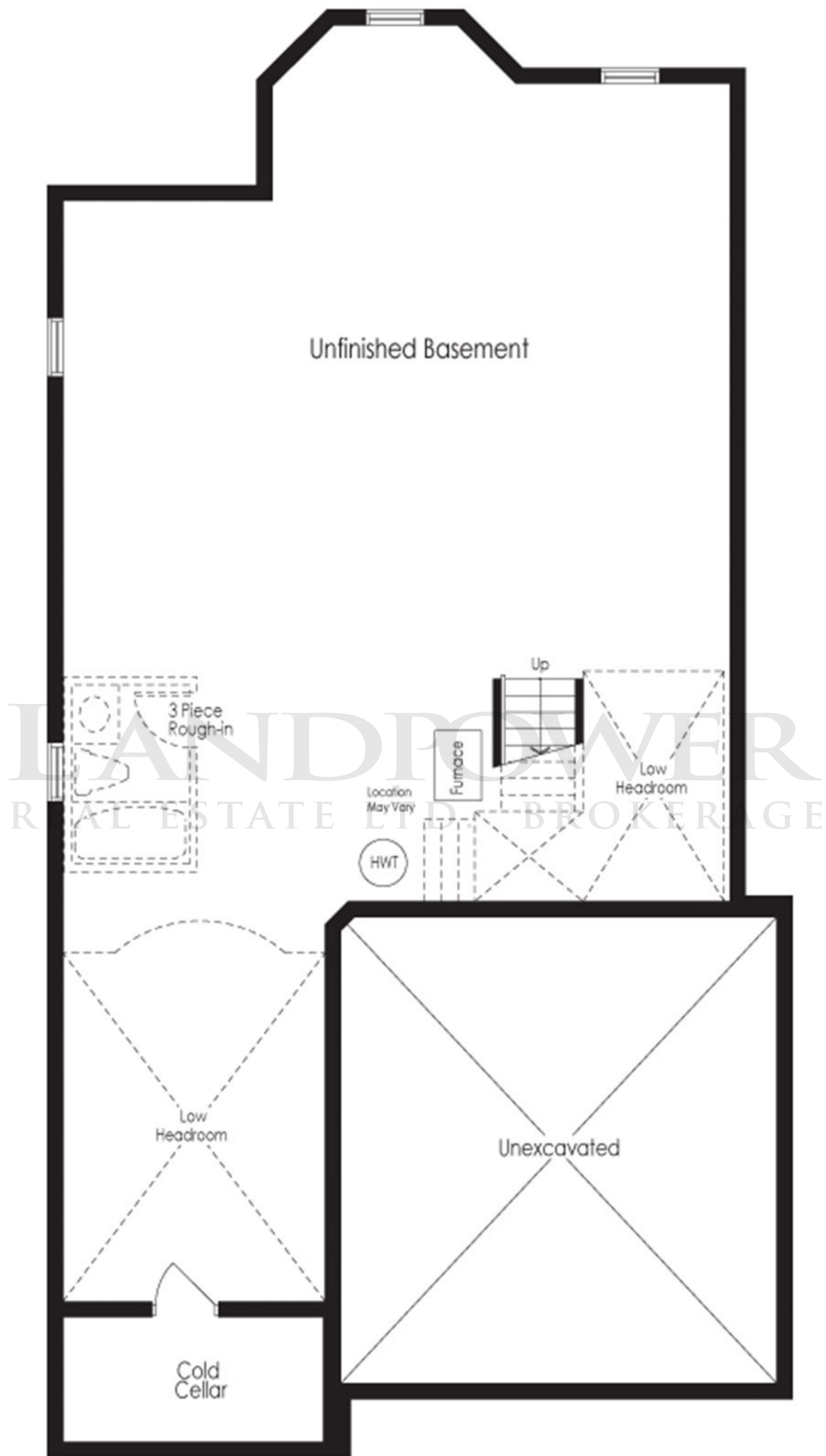
Basement Plan El.'a' & 'B'
