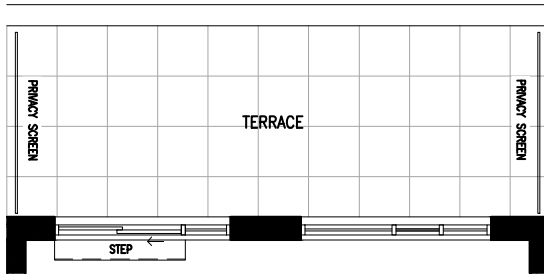
UNIT 328
